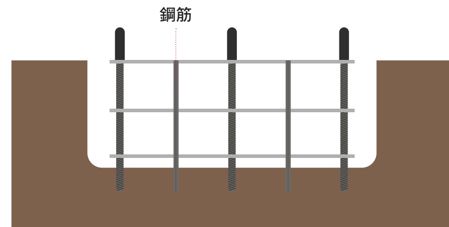
3. 將模板置入其中，並插入數根鋼筋加以固定。
